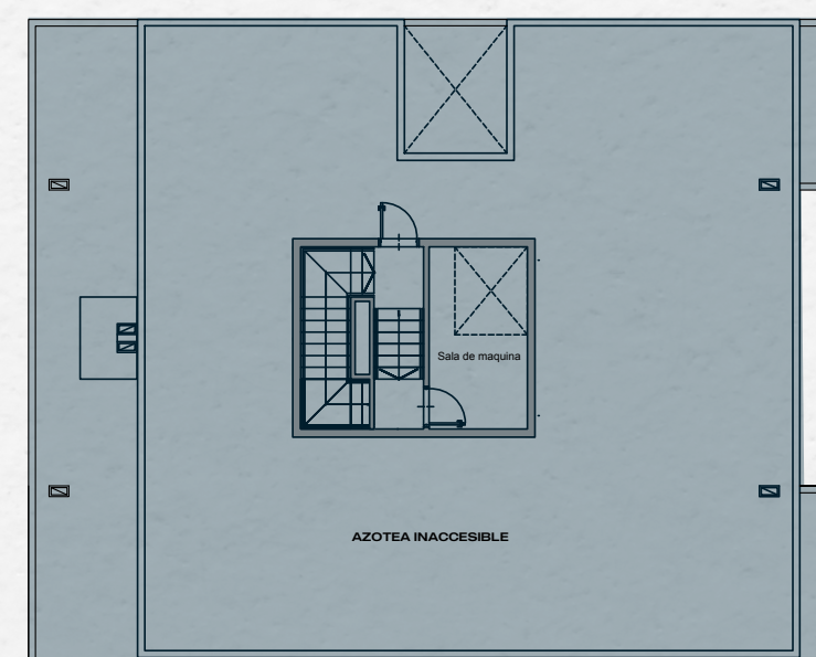
TORRE FRENTE
