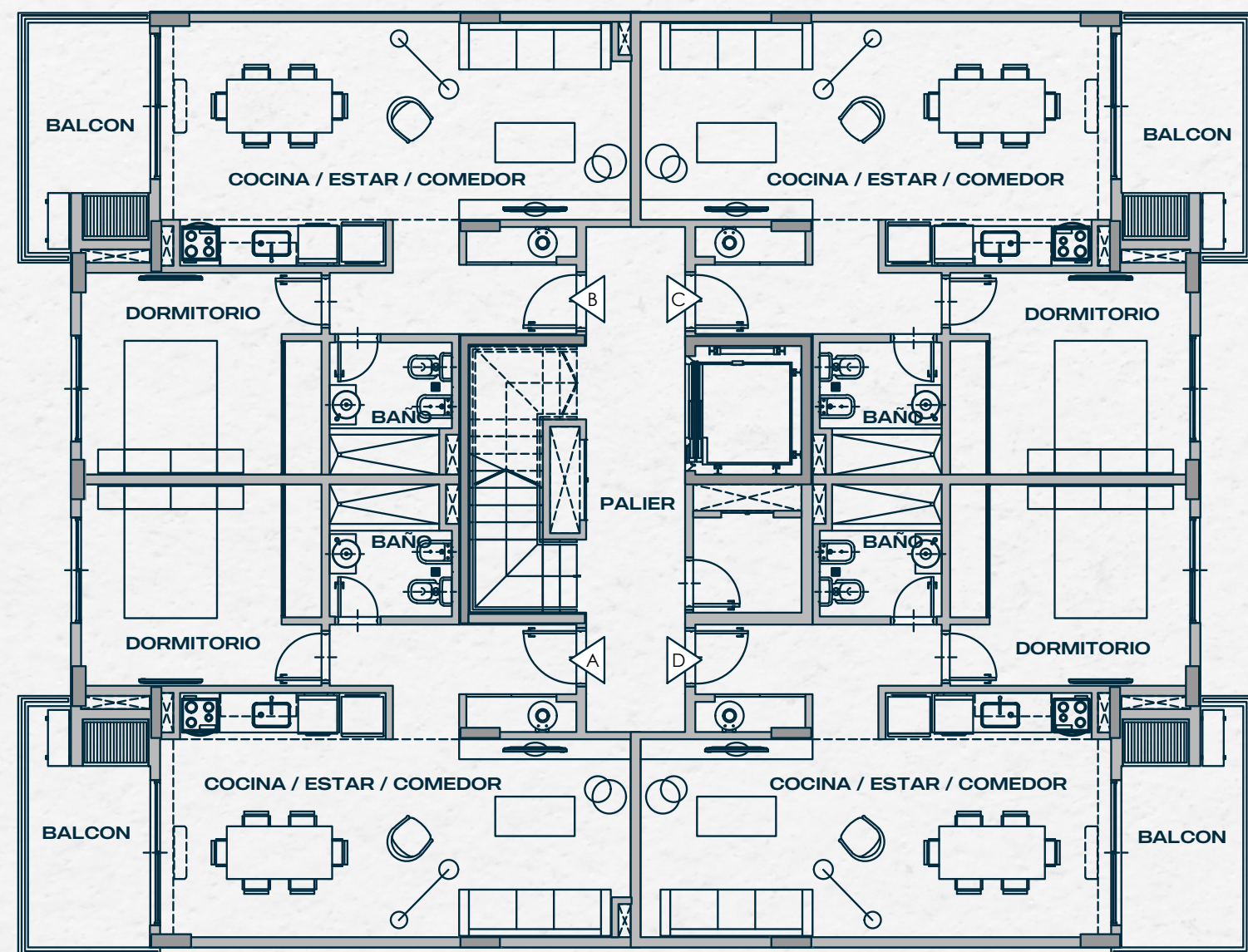
TORRE FRENTE
