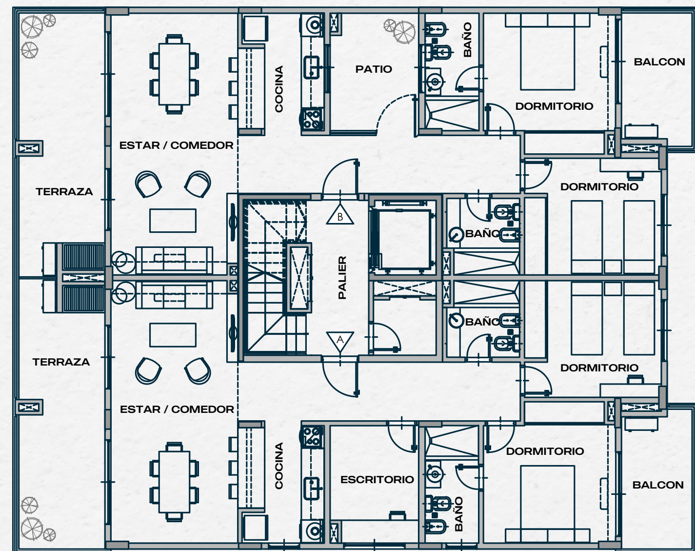
TORRE FRENTE
